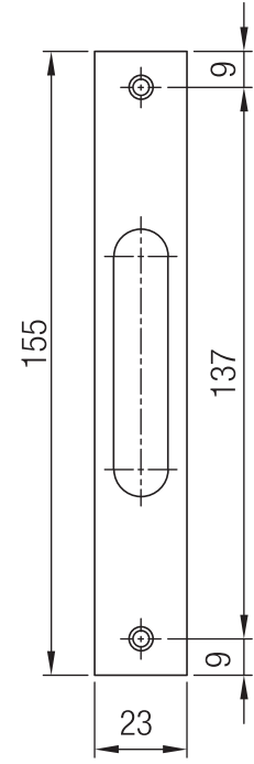
Karşılık Kalınlık: 1,5 mm Striking plate Thickness: 1,5 mm
