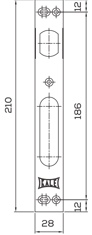
Karşılık Kalınlık: 2,5 mm Striking plate Thickness: 2,5 mm
